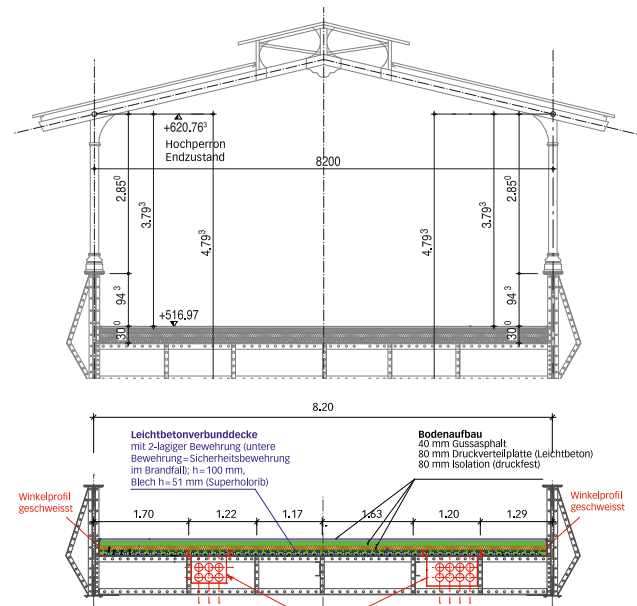
Querschnitt Hochperron (oben) und neuer Bodenaufbau (unten).
